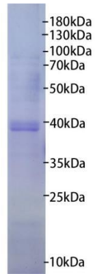
Figure1. SDS-PAGE
